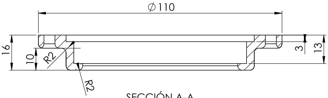
SECCIÓN A-A ESCALA 1 : 1
