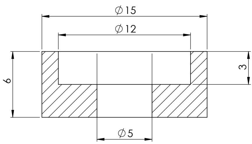
SECCIÓN A-A
