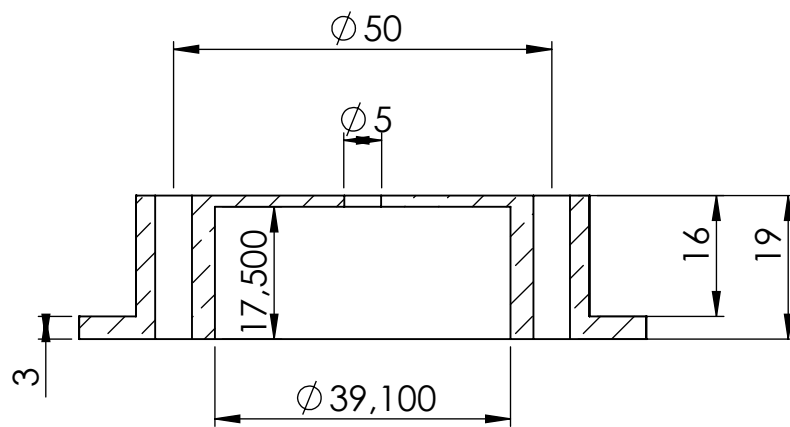
SECCIÓN A-A
