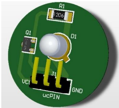
Figura 13 – Montaje del emisor
