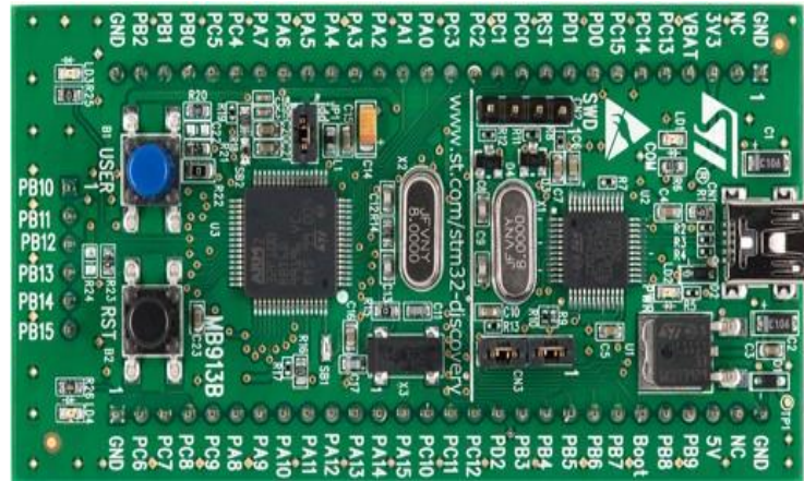
Figura 6 - Placa STM32VLDISCOVERY
