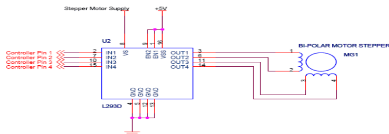
Figura 7 – Montaje de prueba
