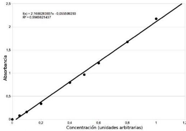
Figura 3 – Curva de absorbancia para soluciones de permanganato de potasio
