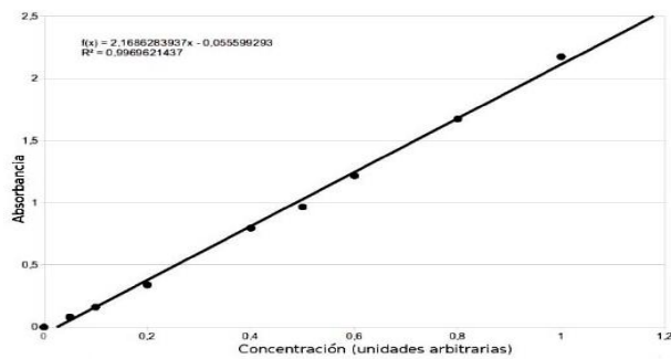
Figura 3 – Curva de absorbancia para soluciones de permanganato de potasio
