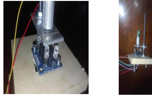
Figura 8 – Montaje de prueba
