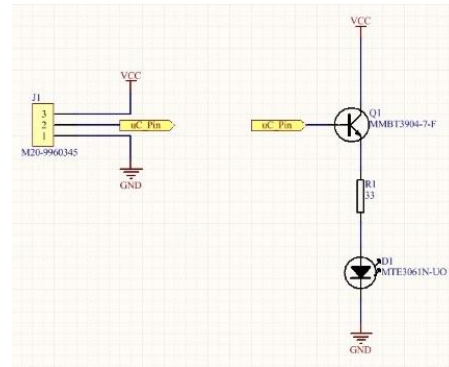
Figura 13 – Montaje del emisor
