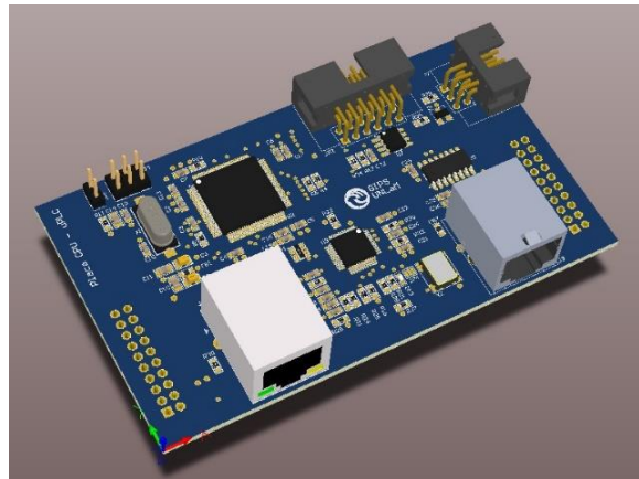
Figura 11 – Placa de control
