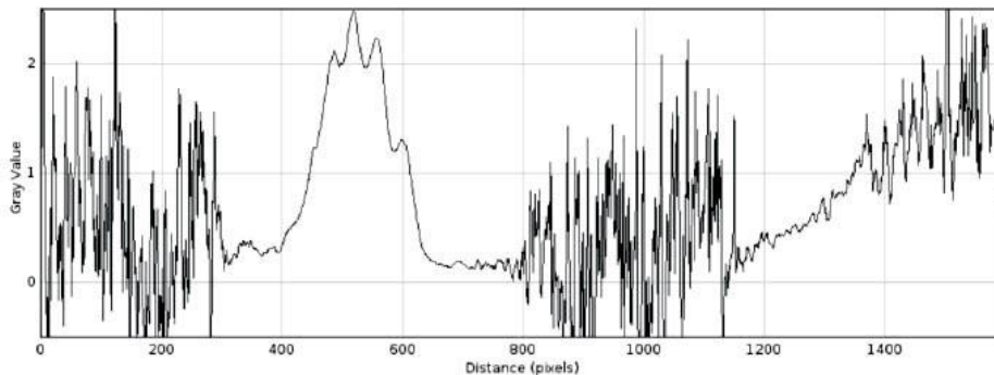
Figura 1 – Espectro de absorción obtenido para una solución diluida de permanganato de potasio
