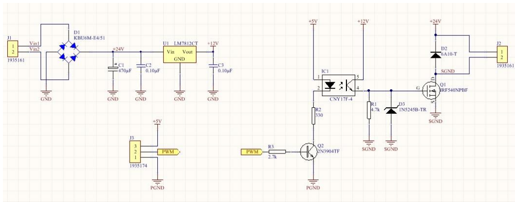
Figura 10 – Esquema de control
